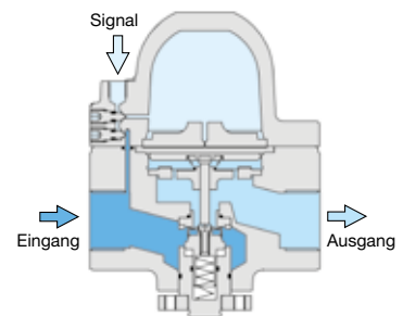
Schnittbild
